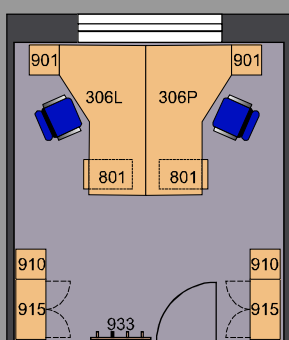
Půdorys varianta 10
