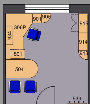
Půdorys varianta 9
